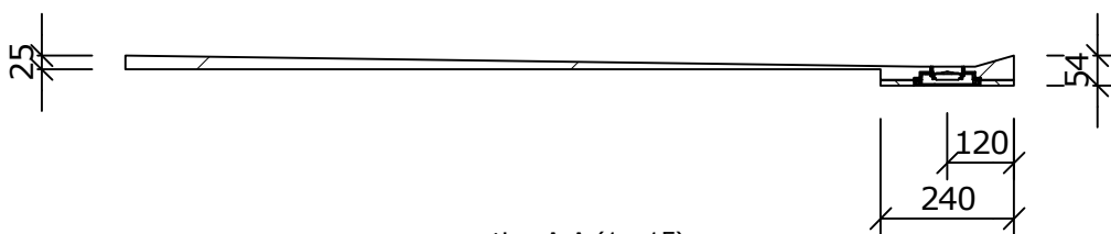
section A-A ( 1 : 15 )
